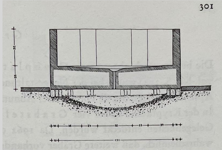
Abb. 3– Schnitt durch das Taufbecken und Sakrarium (Bild: Kubach, Haas „Der Dom zu Speyer“, 1972)
